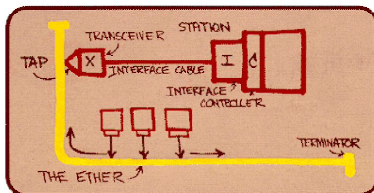
Slika 3: 1972 – ETHERNET
