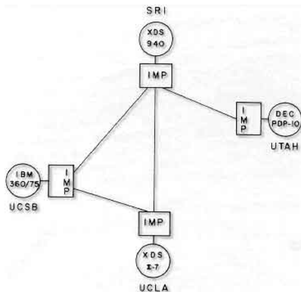
Slika 1: 1969 – začetki ARPANETA
