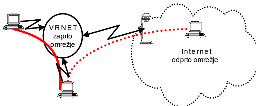
Slika 4: 1994 – VRNET
